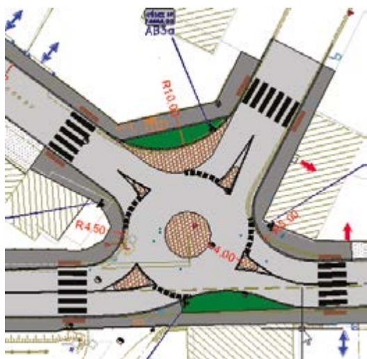
Plan de mise en place du giratoire surélevé
